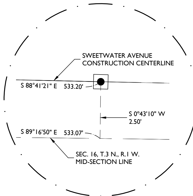
DETAIL N.T.S.
